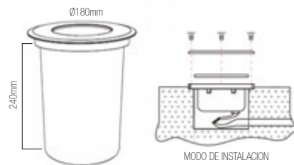
SPOT PISO CILINDRO ACERO 100-240v
