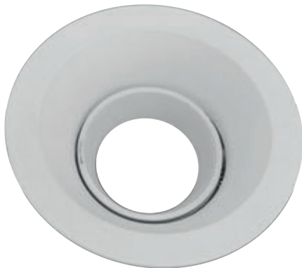
OJO DE BUEY Dirigible GU10 PROFUNDO REDONDO / ALUMINIO Diámetro: Ø105mm Profundidad: 85mm Ref.: Q903-AD
