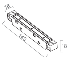
CONECTOR PARA RIEL MAGNÉTICA 48 Ref.: T22A03 Cod.: 010965
