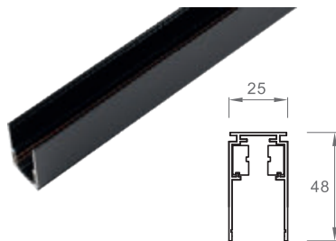
RIEL MAGNÉTICA SOBREPUESTA NEGRA / Aluminio Ref.: T2210A
