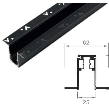
RIEL MAGNÉTICA EMPOTRABLE NEGRA / Aluminio Ref.: T2210C
