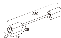
CONECTOR FLEXIBLE PARA RIEL MAGNÉTICA TIPO PERFIL 48v Ref.: T23U05 Cod.: 010918
