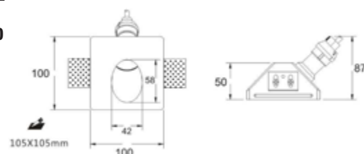
OJO DE BUEY EMPOTRABLE GU10 PINHOLE REDONDO (CON MUELLES DE METAL PARA EMPASTAR EN GYPSUM, ESTUCO O PARED) MR11
