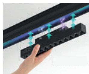
LÁMPARA MAGNÉTICA 18 LUCES / 18W / 3K / 24° Aluminio + ABS 330*23*43mm
