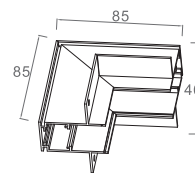
CONECTOR EN L 90° VERTICAL EMPOTRABLE PARA RIEL MAGNÉTICA Ref.: T2206L Cod.: 010970
