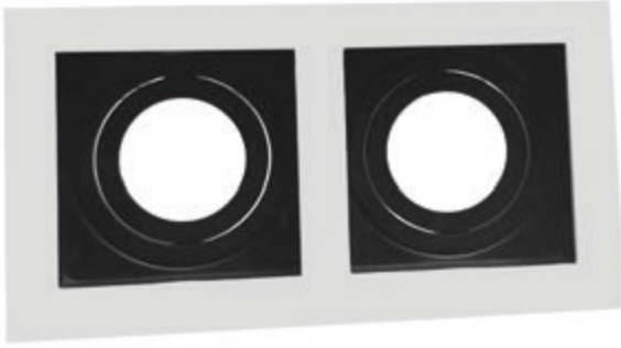
OJO DE BUEY Dicroico 2L / GU10 ALUMINIO / Dirigible (Con Rejilla) Medidas: 190*100mm Ref.: T24-2F BLANCO + NEGRO
